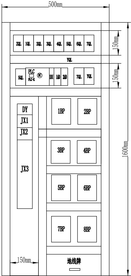
正面内部布置图 1600×500
